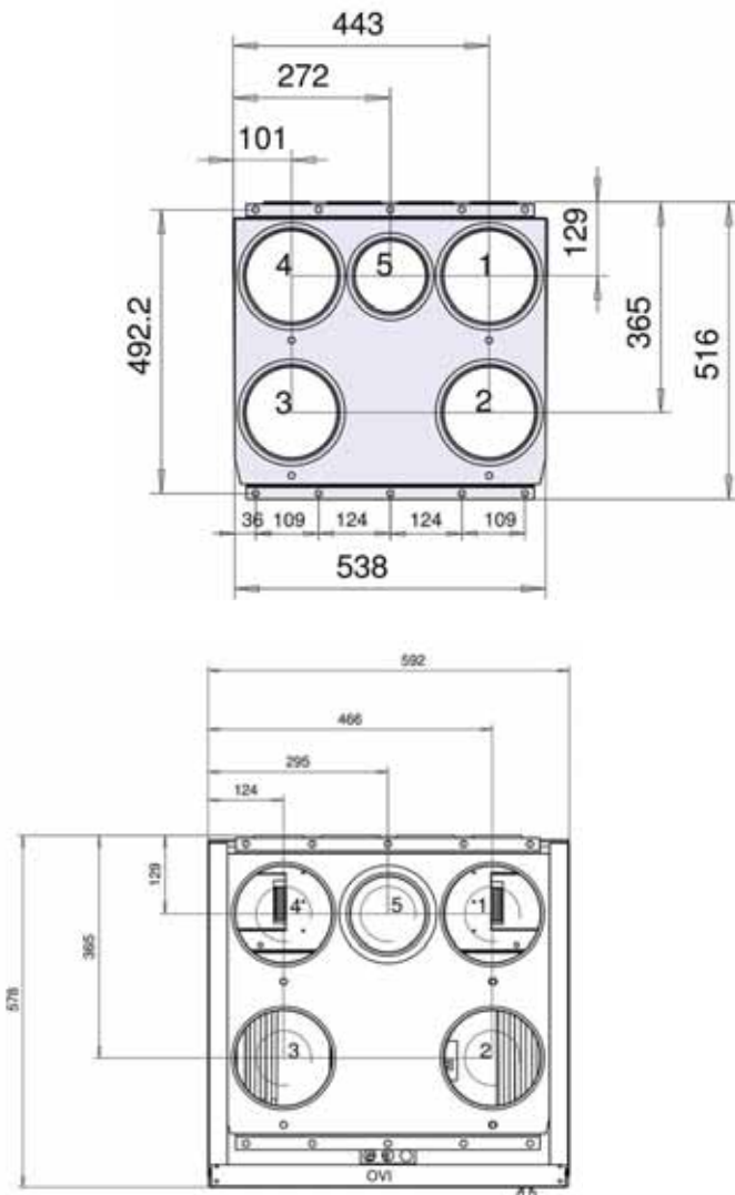
ASENNUSLEVYN MITAT
