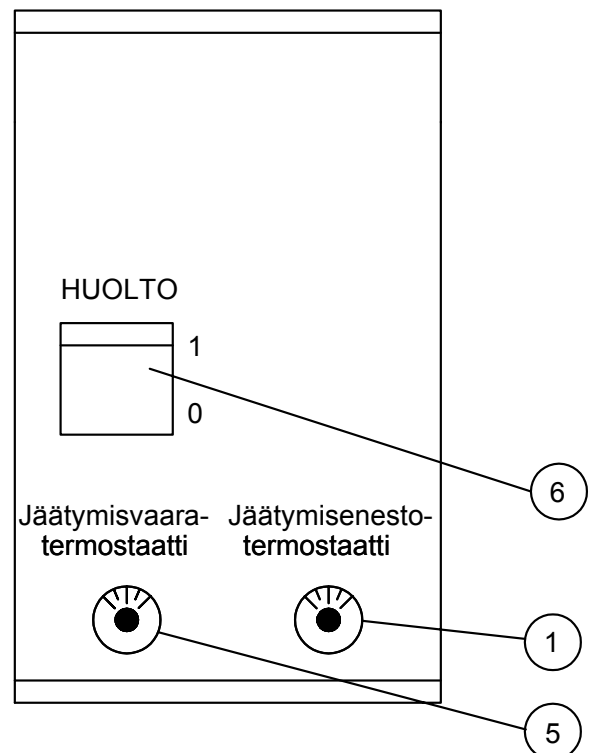
Kuva 2. Ohjainpaneeli ECO 130V
