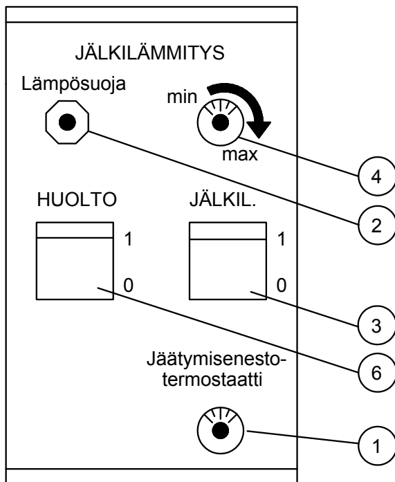
Kuva 1. Ohjainpaneeli ECO 130S
